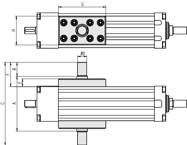
T90、T130、ECT90、ECT130用耳轴套件
