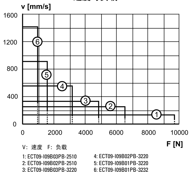
速度与负载
