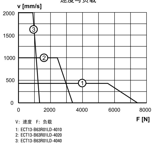
速度与负载
