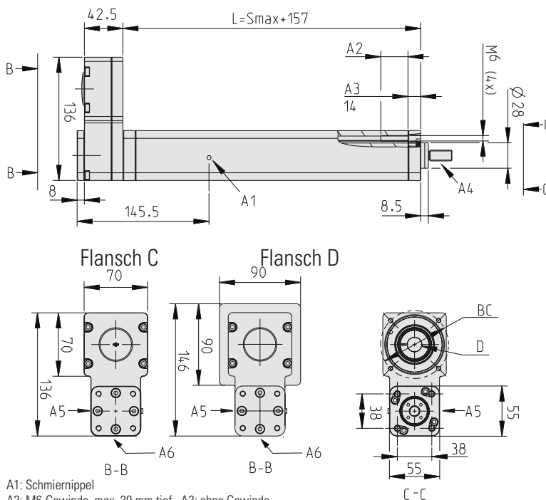
Abmessungen für Parallel-Motoranbau mit RediMount-Flansch
