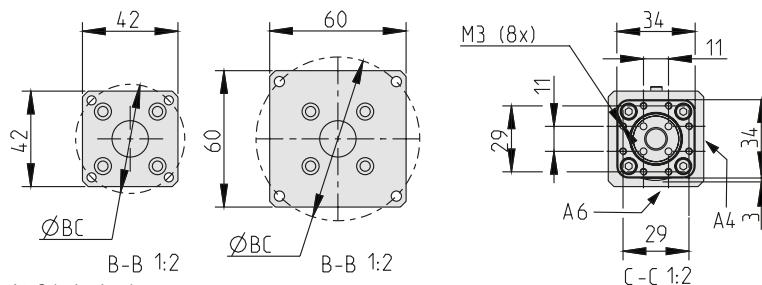
Flansch A
