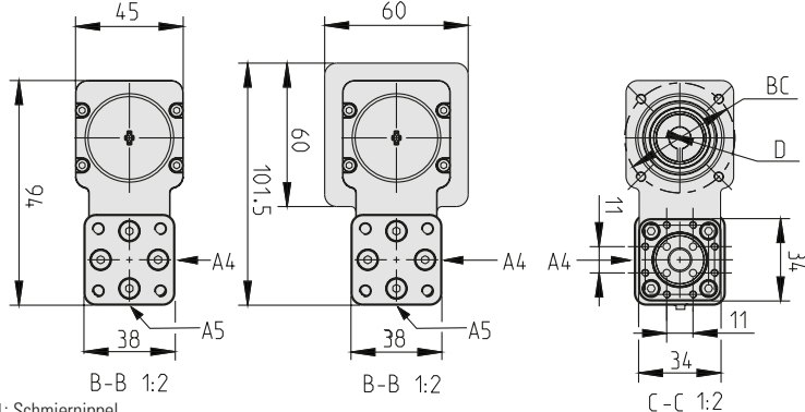
Flansch C
