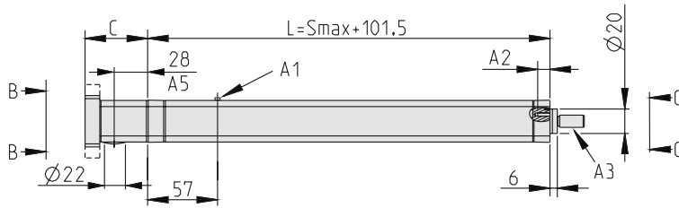
Flansch A
