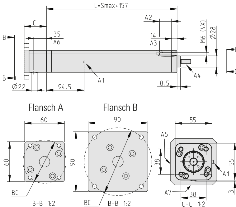
Abmessungen für axialen Motoranbau mit RediMount-Flansch
