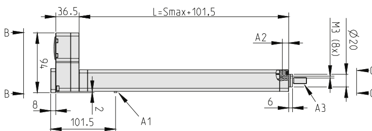
Flansch C
